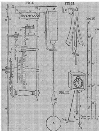
Afb. 11b De verbeterde versie van het slingeruurwerk en zijn mechanisme, getekend door Christiaan Huygens in zijn Horologium Oscillatorium (1673).
