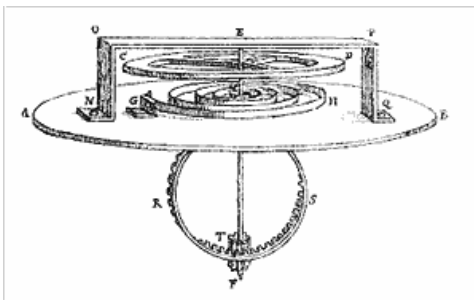
Afb. 11c tekening van een van de eerste springveren van Christiaan Huygens, bevestigd aan een onrust (uitgebalanceerd wielkje), gepubliceerd in zijn brief in het Journal des Sçavants op 25 februari 1675.
