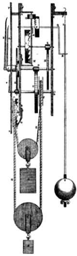
Afb. 11a De klok van Christiaan Huygens uit 1658, beschreven in zijn werk Horologium .
